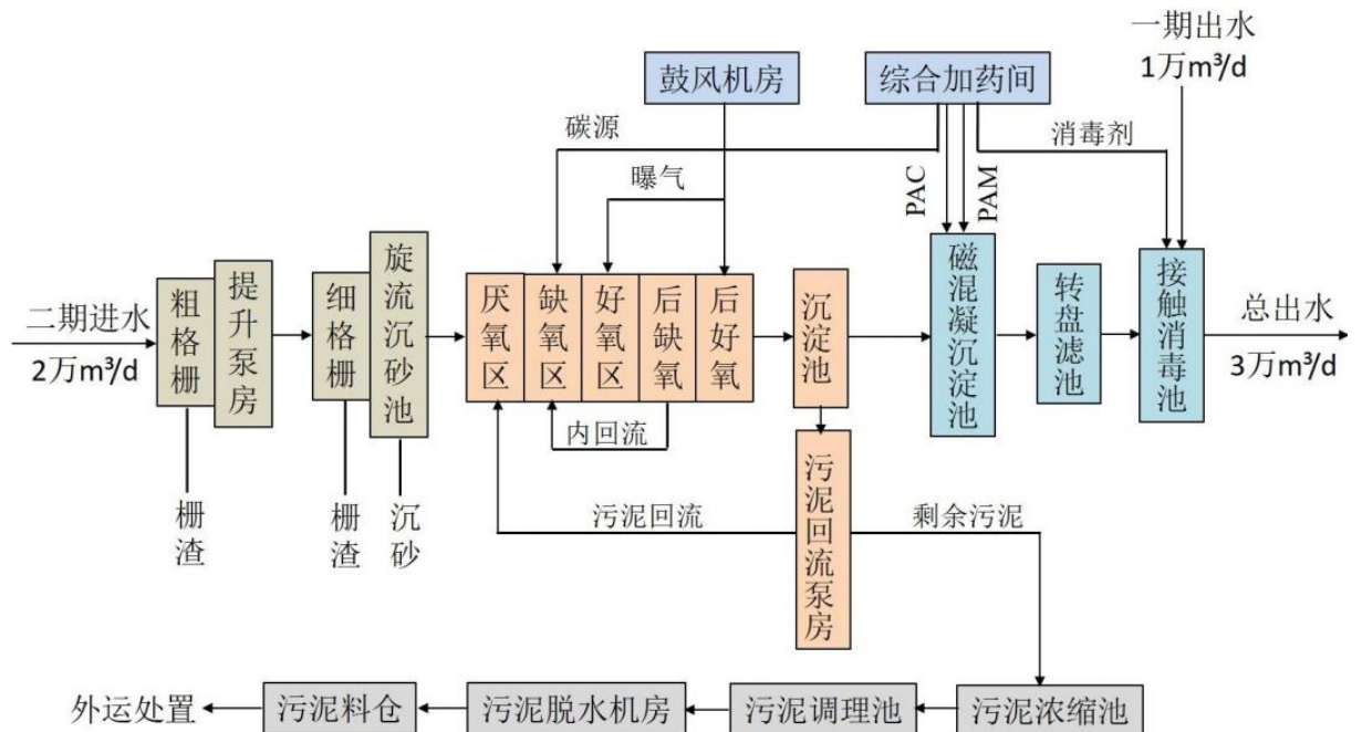
图 4.3-2 巨野河污水处理厂（二期）处理工艺
